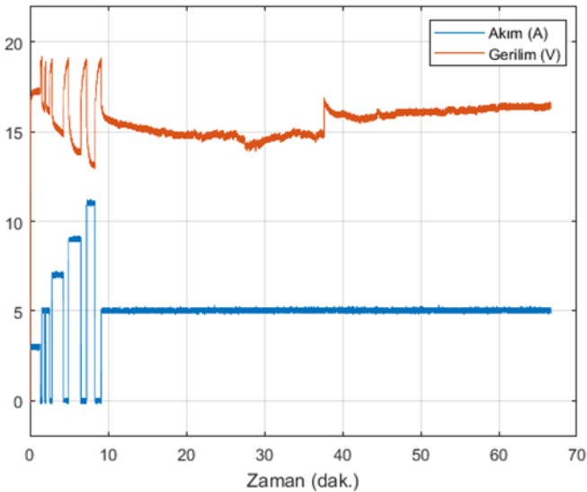
LOX-02 Pili Düşük Sıcaklık (-25°C) Performans Zaman Grafiği
