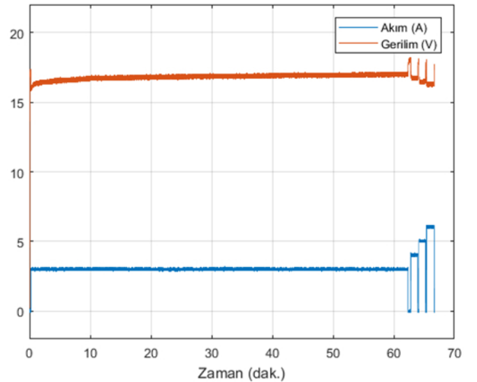
LOX-02 Pili Yüksek Sıcaklık (+25°C) Performans Zaman Grafiği
